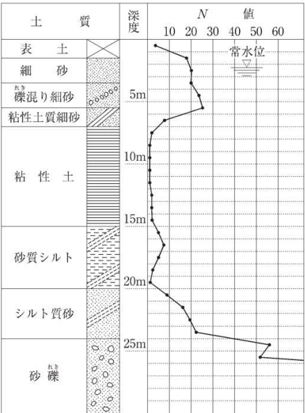
土質柱状図
