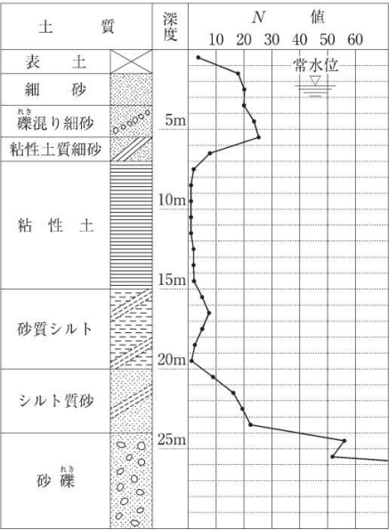
土質柱状図
